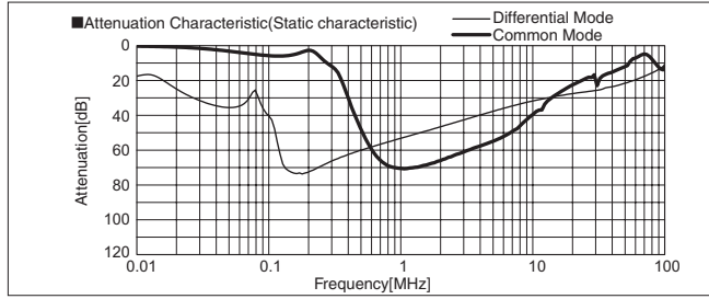
TSC-400-665/TSC-600-665
