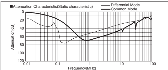
TSD-400-105/TSD-600-105
