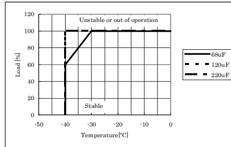
Startup (TUNS100)
